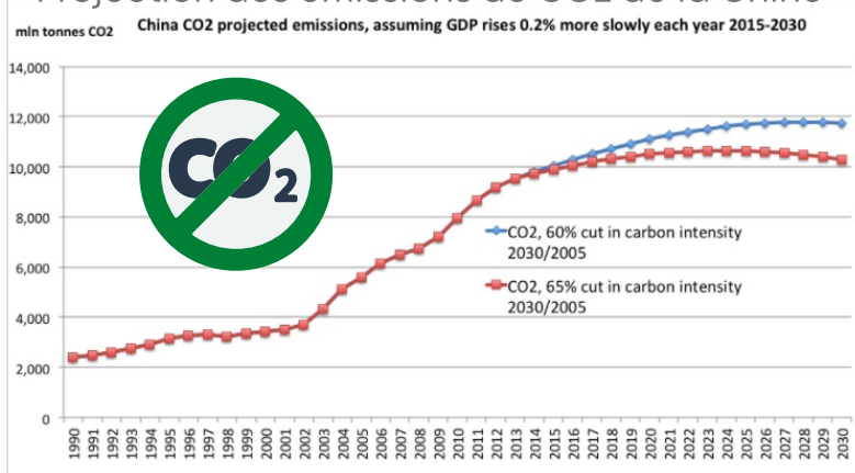
Projection des émissions de CO 2 de la Chine
